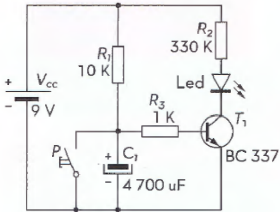
Fig. 4.33. Circuit d'un temporitzador retardat a la connexió
