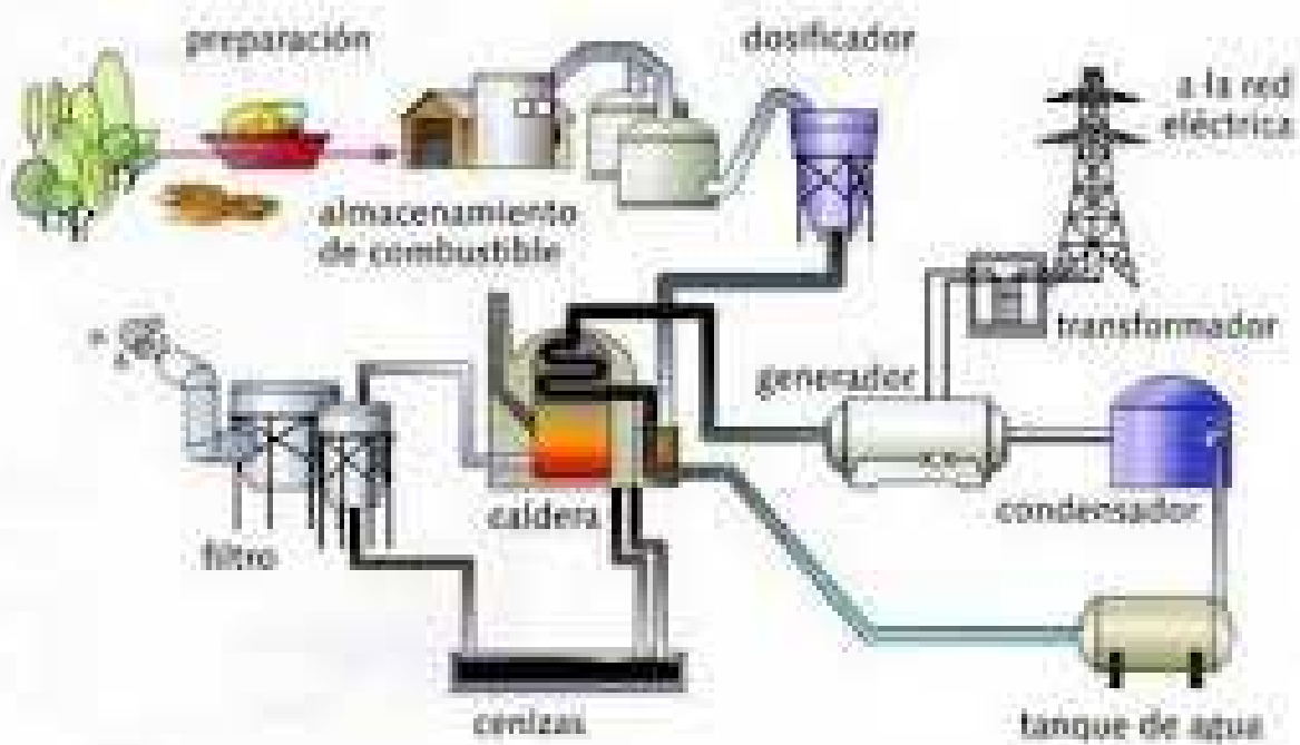
Esquema de una central de biomasa.
