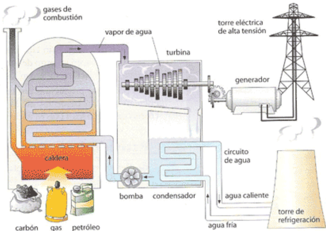
Esquema de una central térmica.
