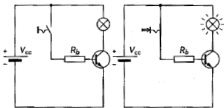
Fig. 4.15. Transistor treballant en commutació. a) Estat obert ( OFF ); b) Estat de conducció ( ON )
