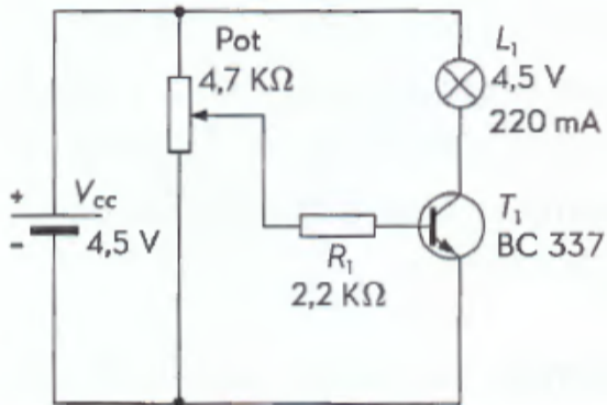
Fig. 4.32. Circuit d'un regulador electrònic, funcionant en mode lineal.
