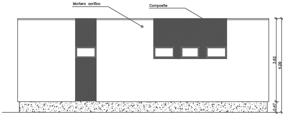
ALZADO LATERAL IZQUIERDO
