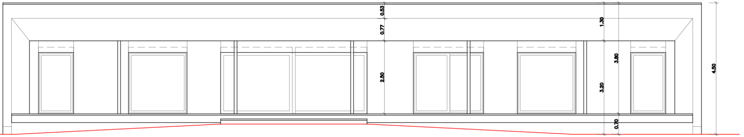
ALZADO TRASERO
