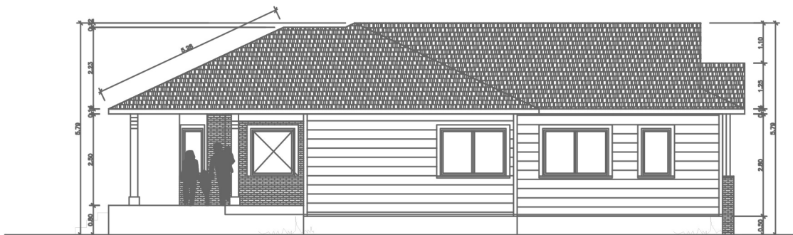
ALZADOS ESTE
