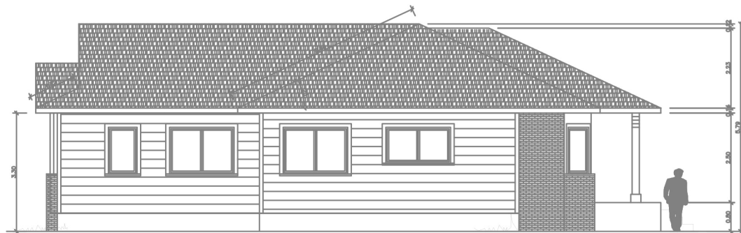
ALZADOS OESTE
