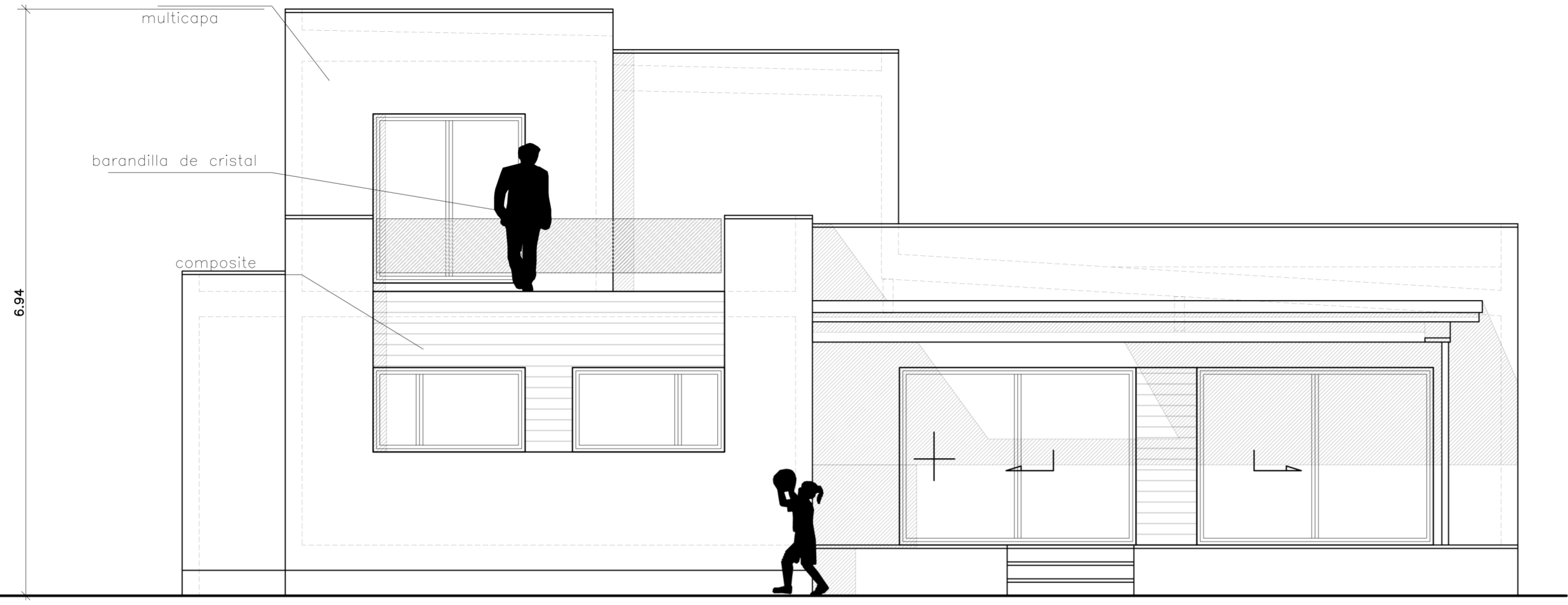
ALZADO OESTE
